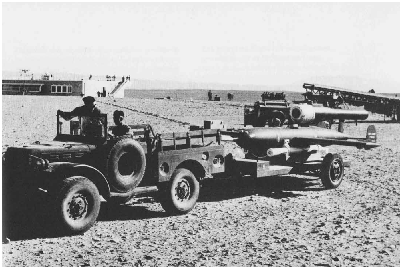
▲ ▼ Les premiers essais, avec l'Arsenal 2501, type VI
