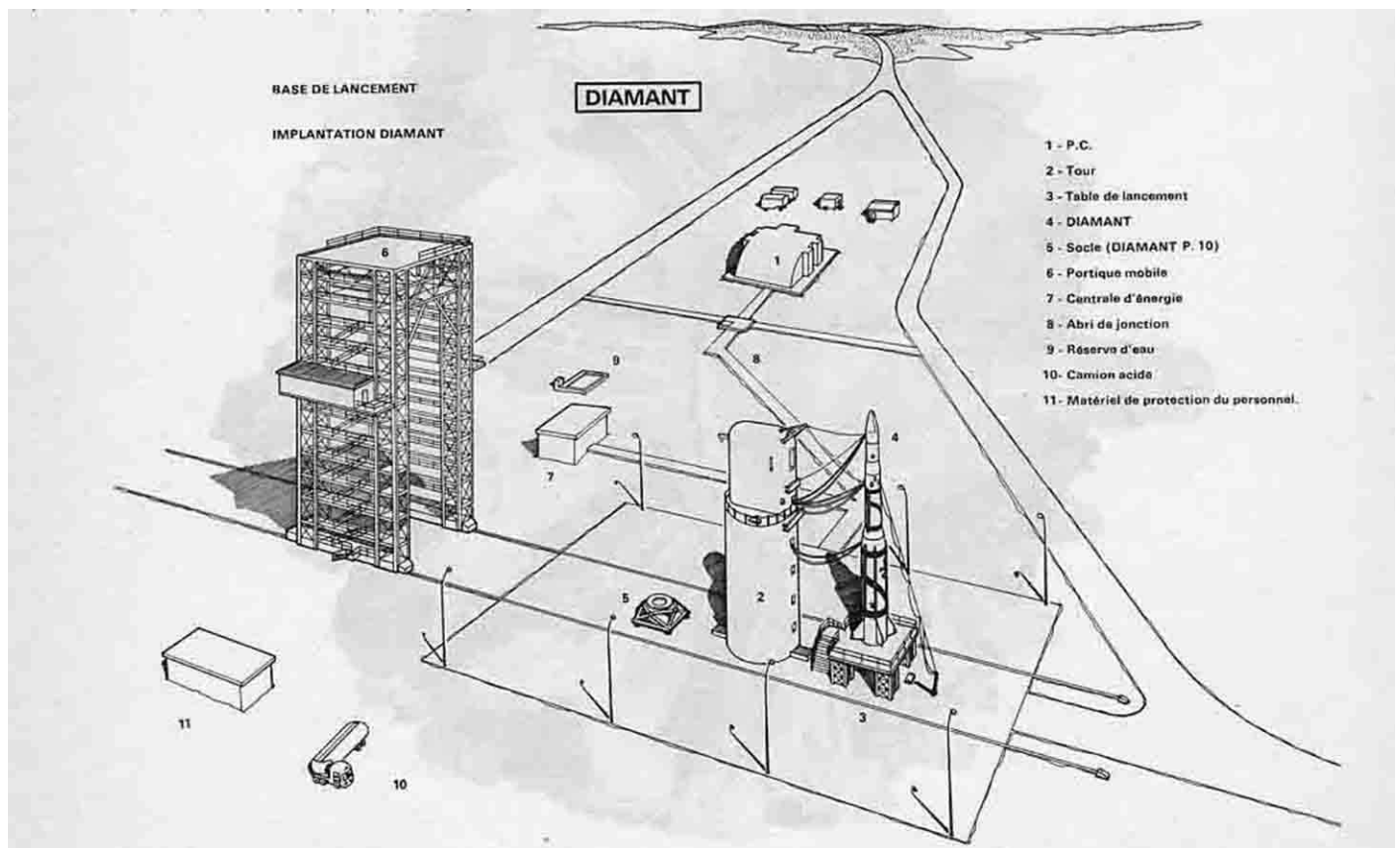
▲ Schéma d'installation de la fusée Diamant
