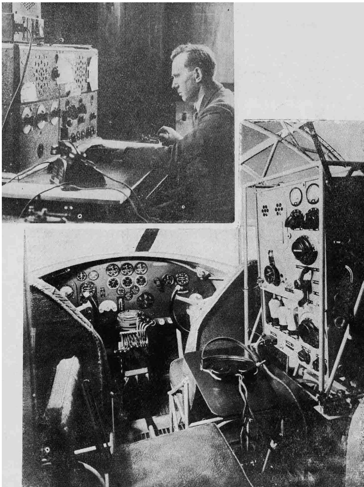
Poste de pilotage et installation radioélectrique d'un Savoia-Marchetti S.73
