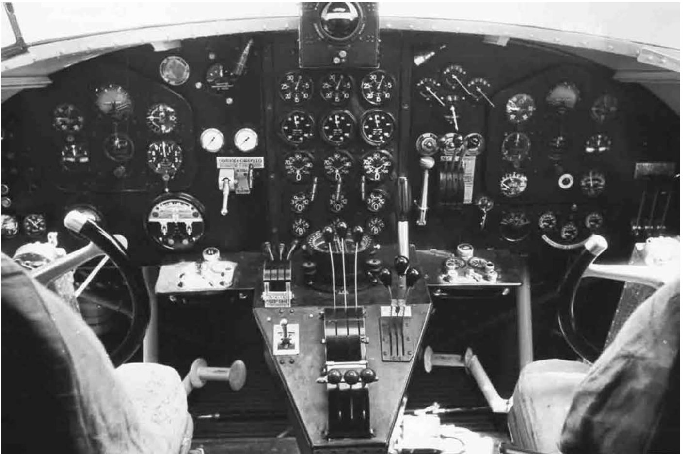
▲ ▼ Poste de pilotage et cabine d'un Savoia-Marchetti S.83
