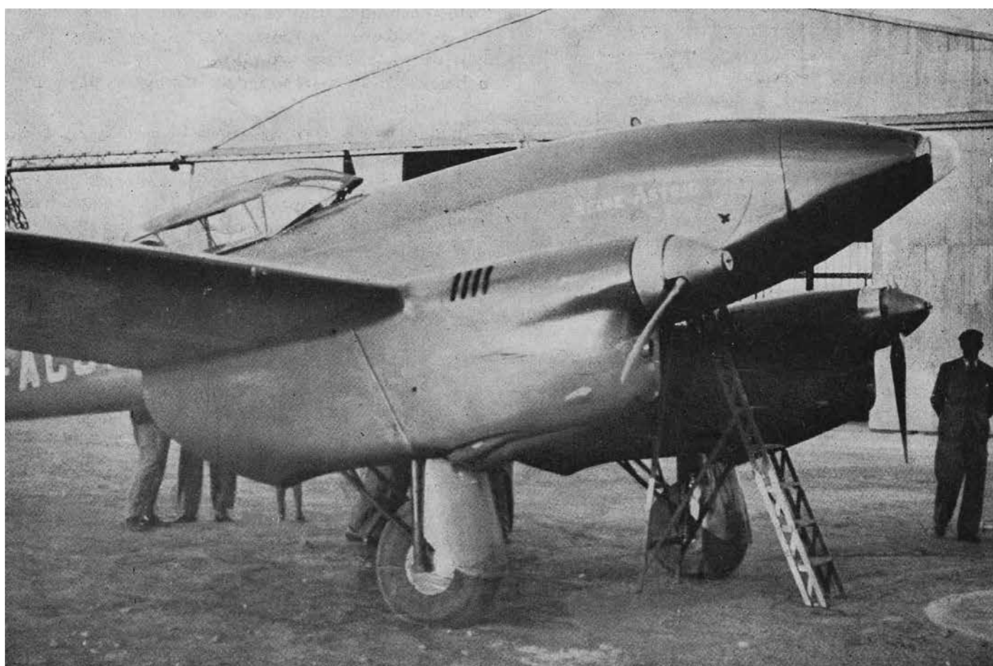
▲ ▼ Le De Havilland DH 88 Comet G-ACSR «Reine Astrid»
