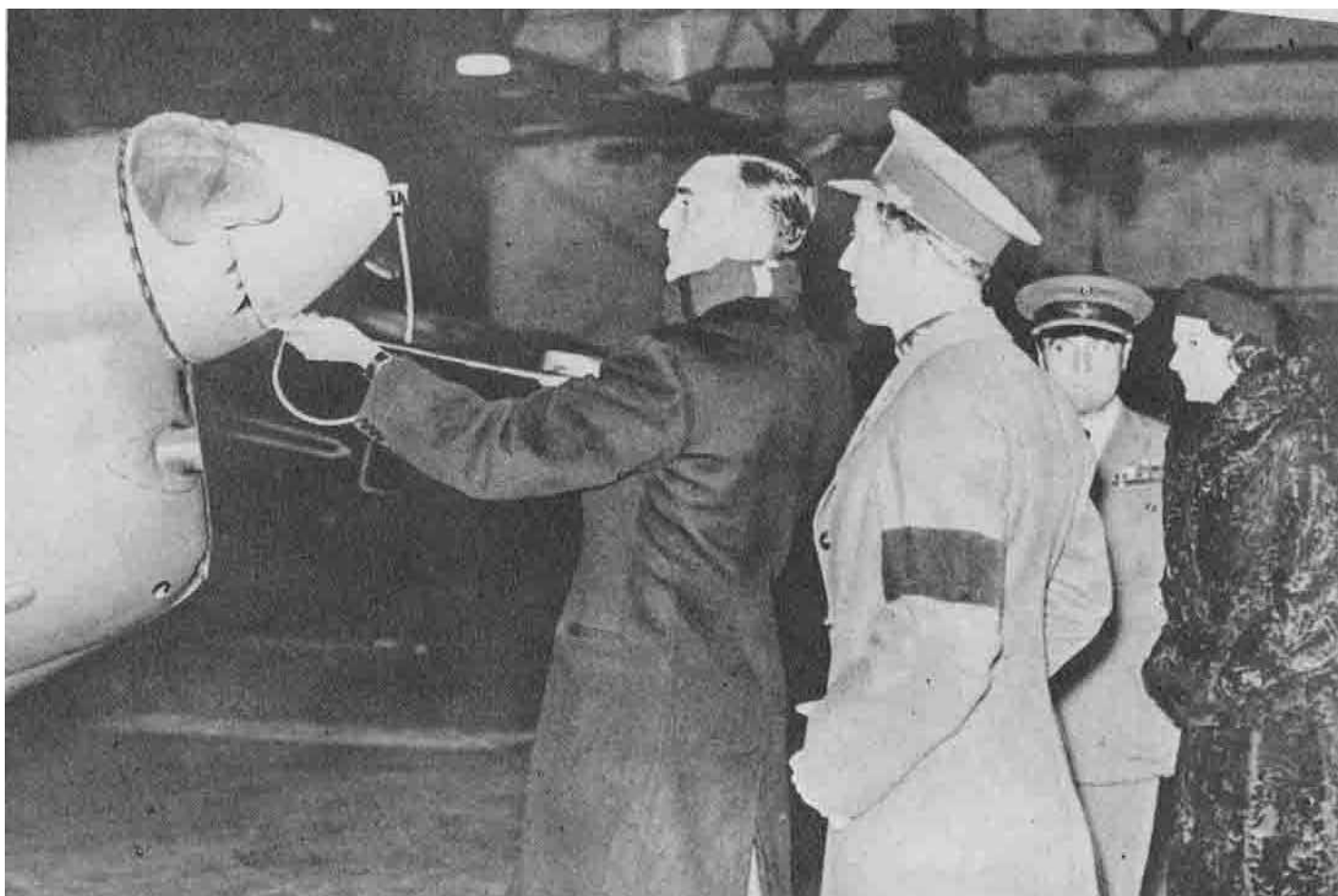
▲ Le roi Léopold s'intéresse au dispositif de "gonflage de l'hélice" qui permet de passer au grand pas après le décollage. La reine Astrid est à droite
