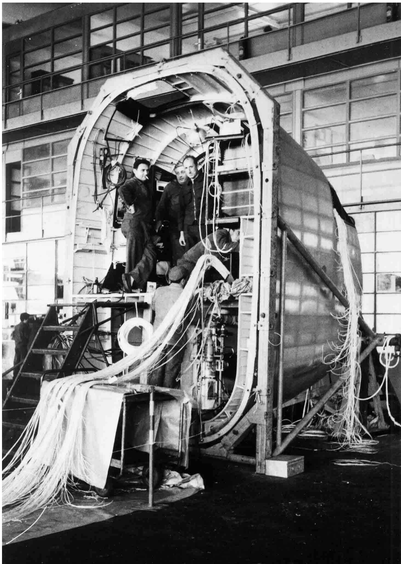
Deux-Ponts dans l'atelier d'Air France à Maison-Blanche
